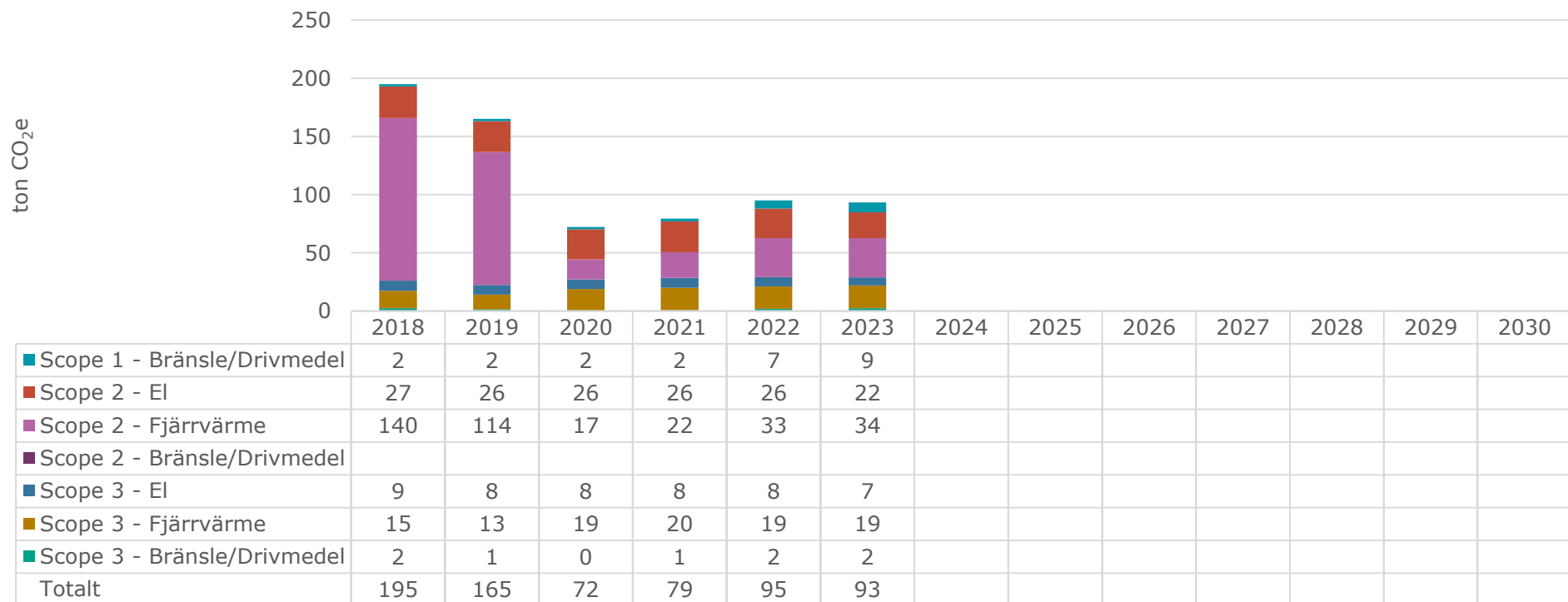
Diagram 4.3 Klimatutsläpp location-based method
