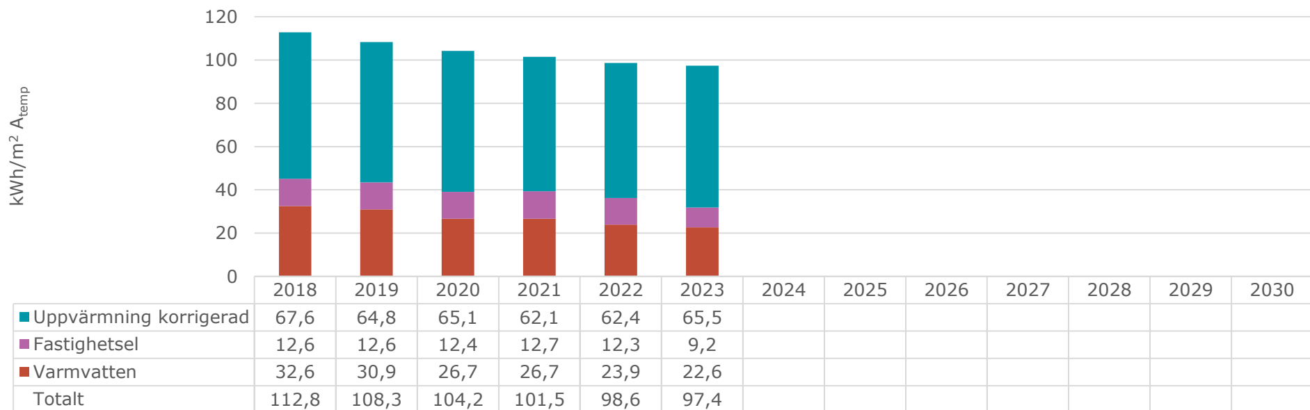
Diagram 2.2 Byggnadernas energiaprestanda uppdelad på uppvärmning, fastighetsel och varmvatten
